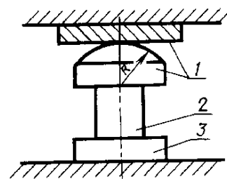
1 и 3 — опоры; 2 — образец
