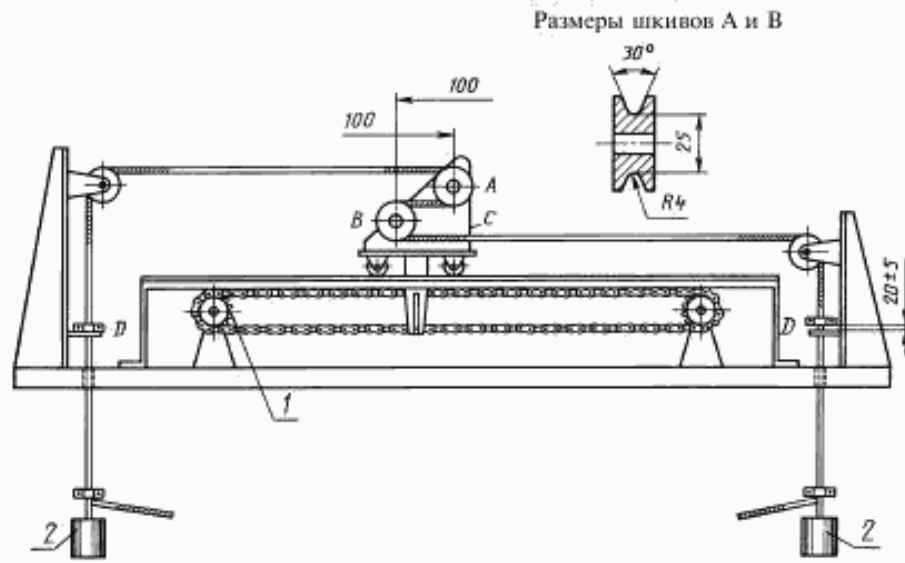
A, B — шкивы; C — салазки; D — сдерживающие зажимы; I — звездочка ( D_{\text{ср}} = 88,9 мм, z = 20 , шаг 12,7 мм); Z — груз массой 0,25 кг
