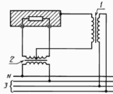
Схема для испытания электрической прочности по п. 13.4
