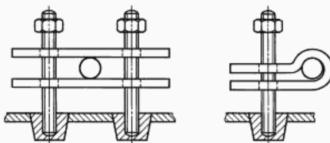
Примеры крепления шнура (допустимые конструкции)
