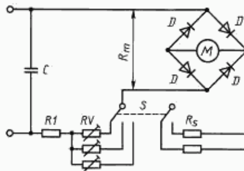
Схема измерения токов утечки
