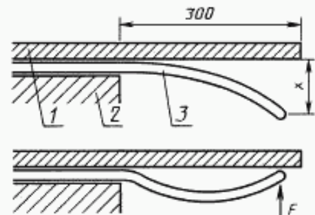
Положение одеяла для испытания на устойчивость к сморщиванию по п. 22.16
