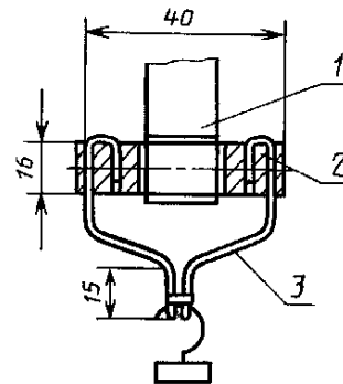
Схема зажимного устройства
