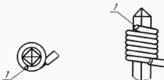
1 — конец накрутки
