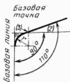
Оптический калибр
