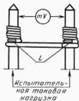
Модифицированные соединения накруткой
