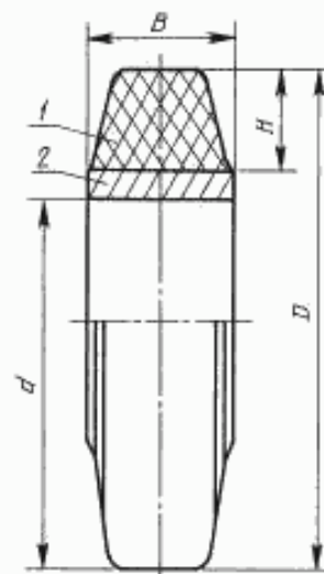
Бандажная массивная шина
