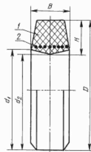
Безбандажная массивная шина с коническим основанием
