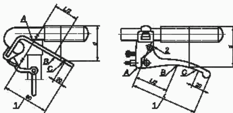
1 — длина рукоятки; 2 — вспомогательный механизм
