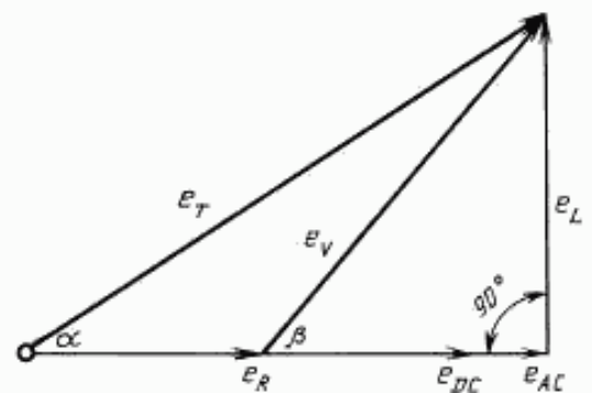
Векторная диаграмма напряжений
