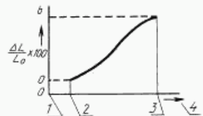
1 — подстроечник удален; 2 — минимальное положение; 3 — максимальное положение; 4 — смещение
