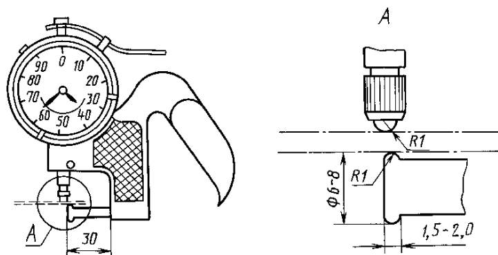
Прибор с круговой шкалой
