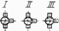
Положение крана 1
