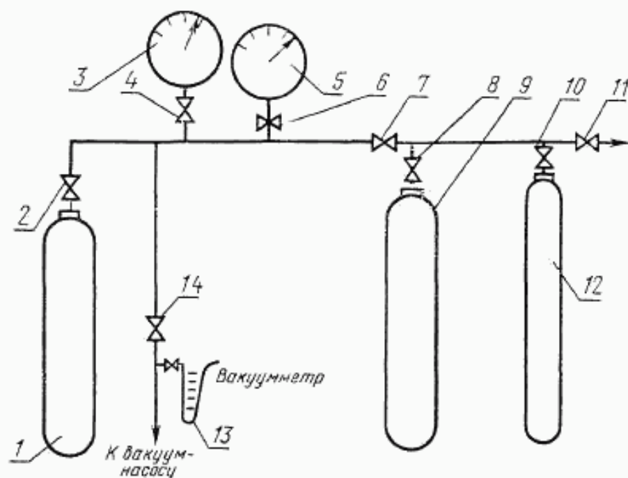
1, 9, 12—баллоны; 3, 5—манометры; 2, 4, 6, 7, 8, 10, 11, 14—вентили; 13—вакуумметр
