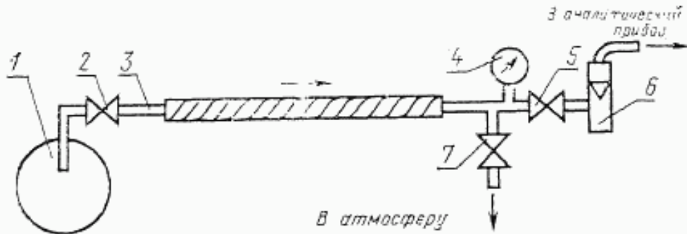
1—заводской трубопровод; 2, 5, 7—вентили; 3—трубопровод для подачи газа к месту анализа; 4—манометр; 5—ротаметр, реометр или другой газовый счетчик
