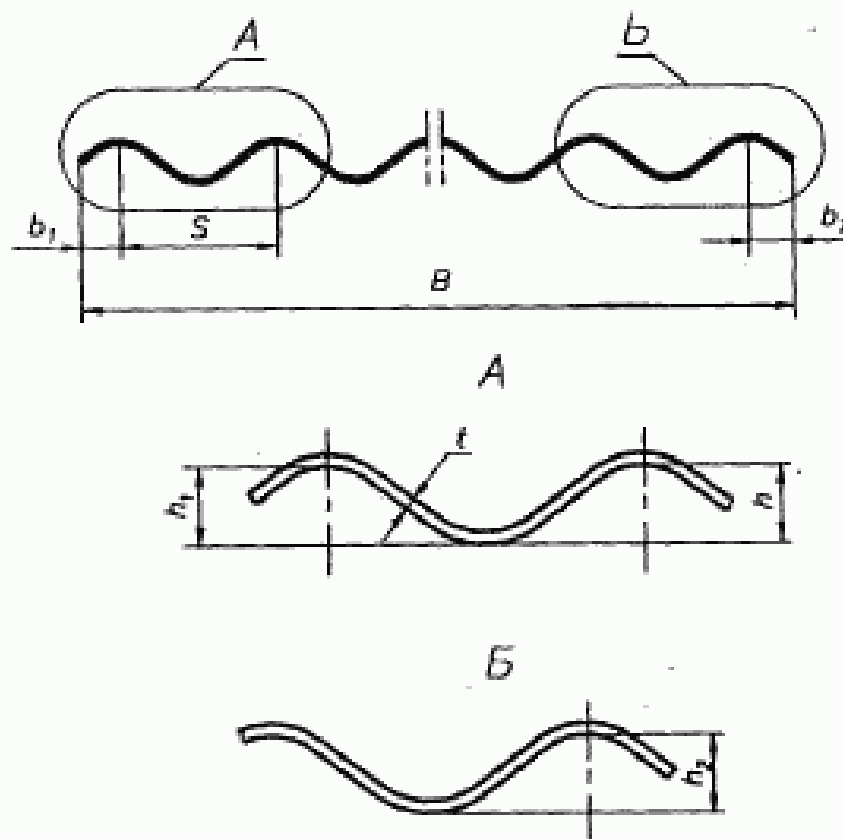
Рисунок 1 — Форма поперечного сечения волнистого листа
