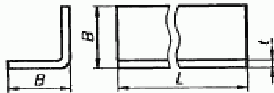
Рисунок 4 — Рамбовая угловая деталь
