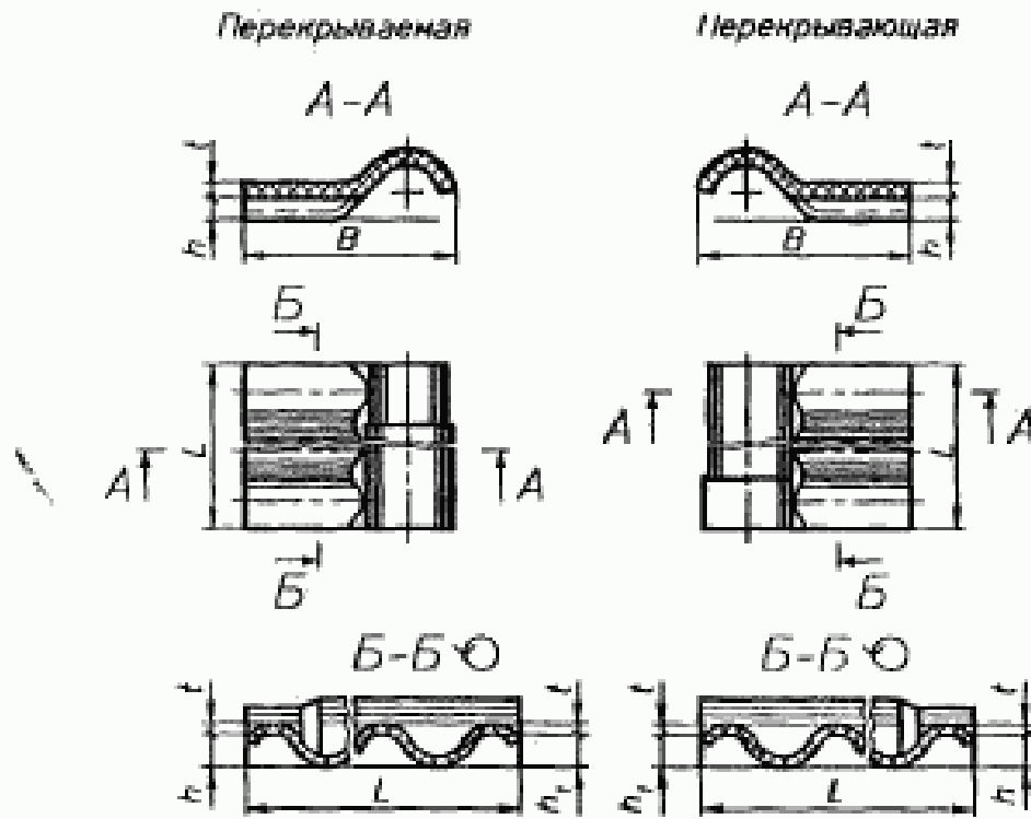
Рисунок 2 — Коньковые детали
