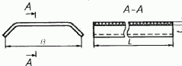
Рисунок 5 — Лотковая деталь
