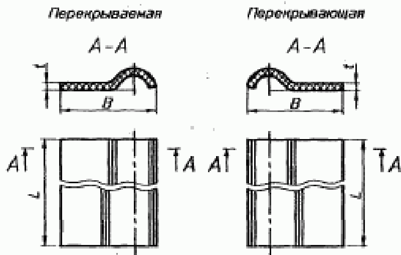
Рисунок 3 — Упрощенные коньковые детали
