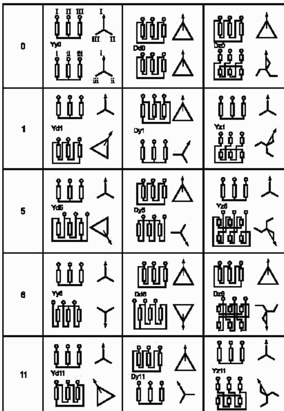
Рисунок Г.1 — Стандартные схемы и группы соединения обмоток
