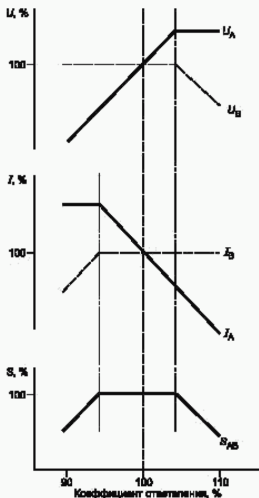
Рисунок 3 — Комбинированное регулирование напряжения (режим a )
