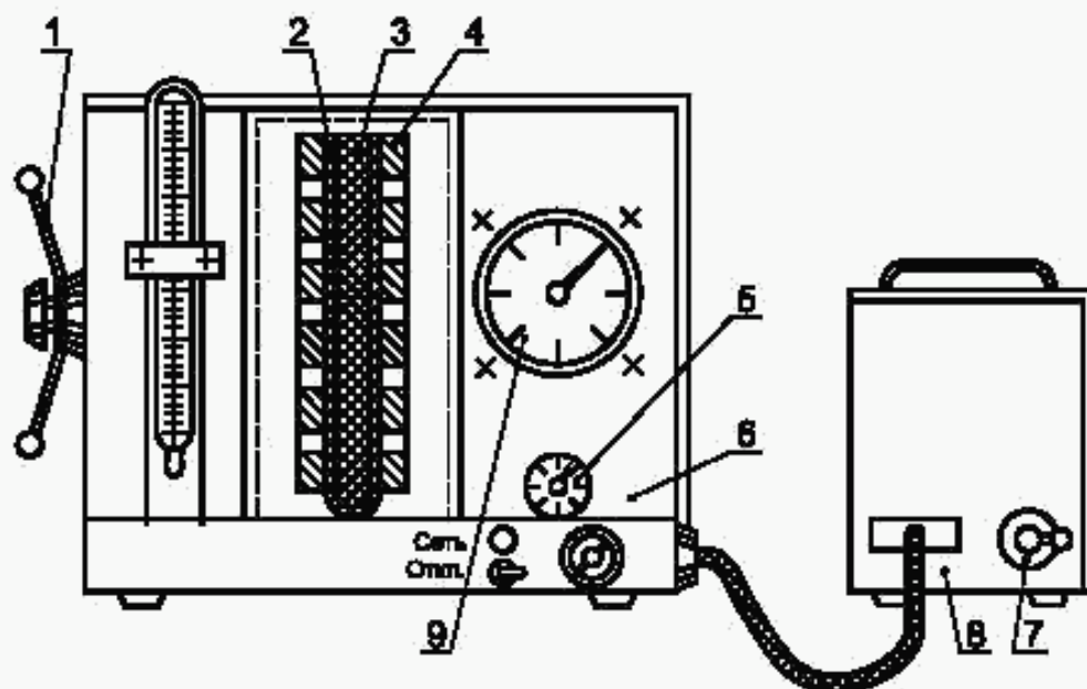
1 — рукоятка; 2 — элементарная проба; 3 — подложка; 4 — подвижная электродная система; 5 — манометр; 6 — датчик; 7 — тумблер; 8 — тереоимметр; 9 — переключатель диапазонов
