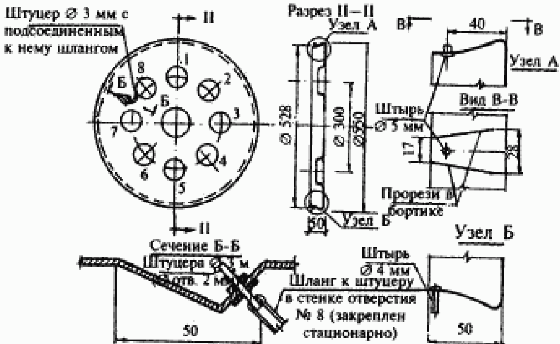
Рисунок 4 — Пластина с отверстиями к кожуху вентилятора
