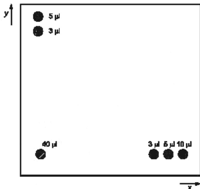
Рисунок 1 — Двухнаправленная тонкослойная хроматография
