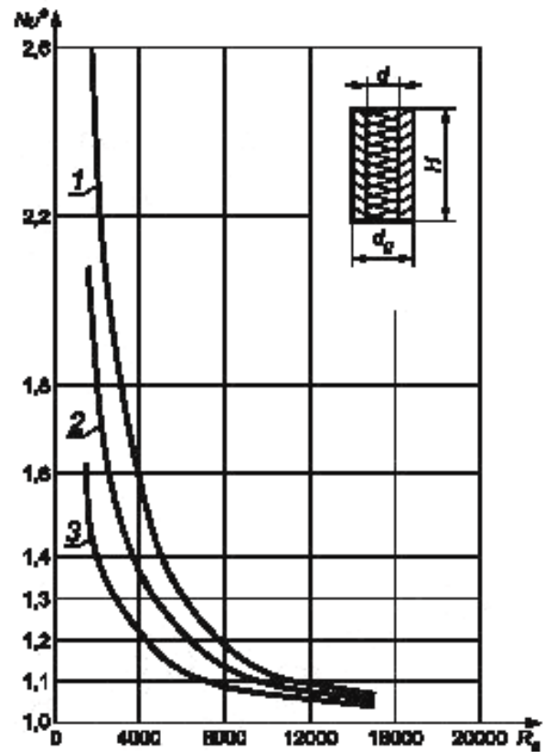
Рисунок А.5 — Диаграмма для теплоизоляционной системы общей толщиной d_g = 0,30 м
