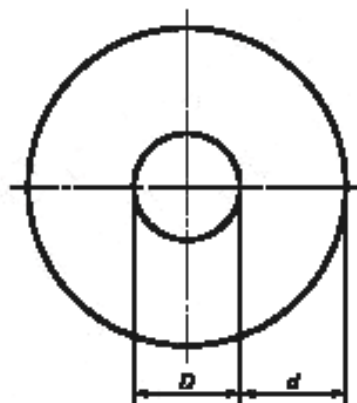
Рисунок А.2 — Схема сжатия теплоизоляции труб
