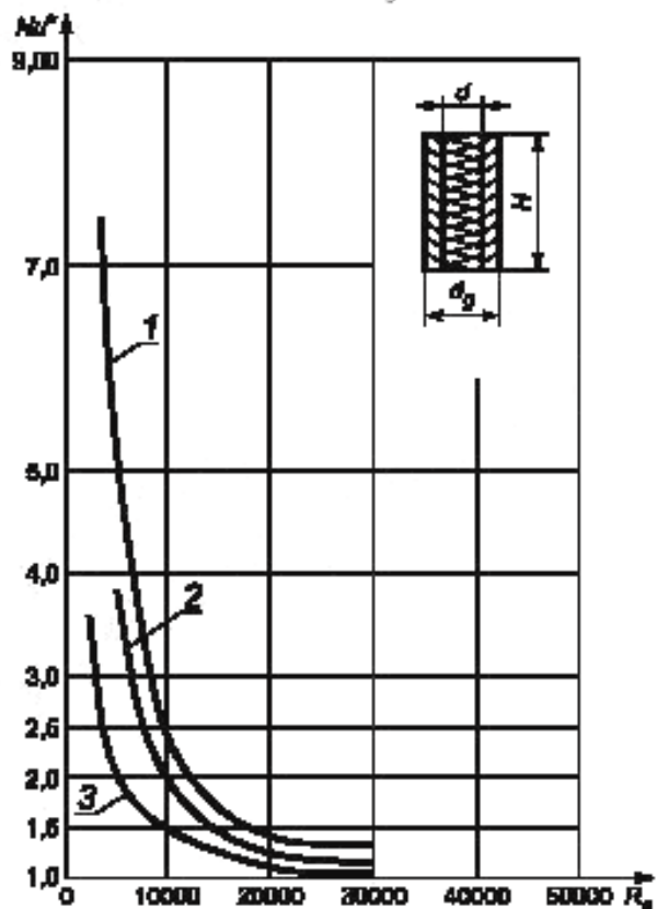
Рисунок А.6 — Диаграмма для теплоизоляционной системы общей толщиной d_g = 0,60 м
