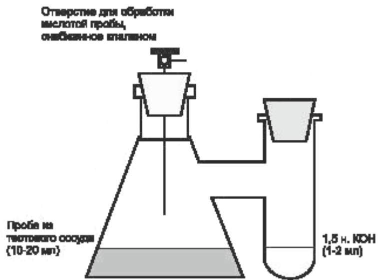
Рисунок А.3 — Система для улавливания растворенного ^{14}\text{CO}_2
