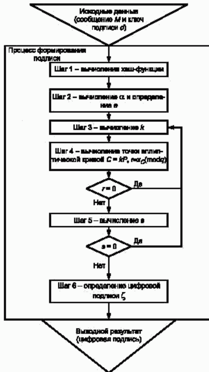
Рисунок 2 — Схема процесса формирования цифровой подписи
