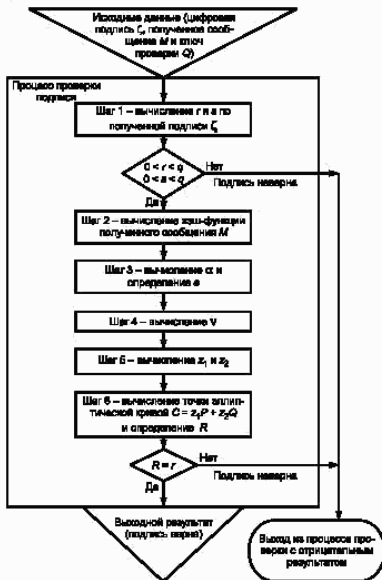
Рисунок 3 — Схемa процесса проверки цифровой подписи
