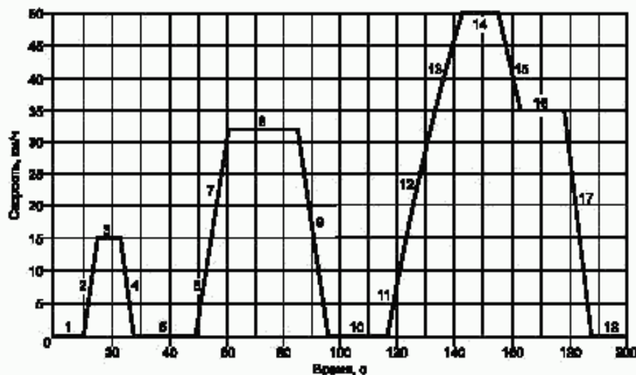
Рисунок 2 — Простой городской цикл (195 с)
