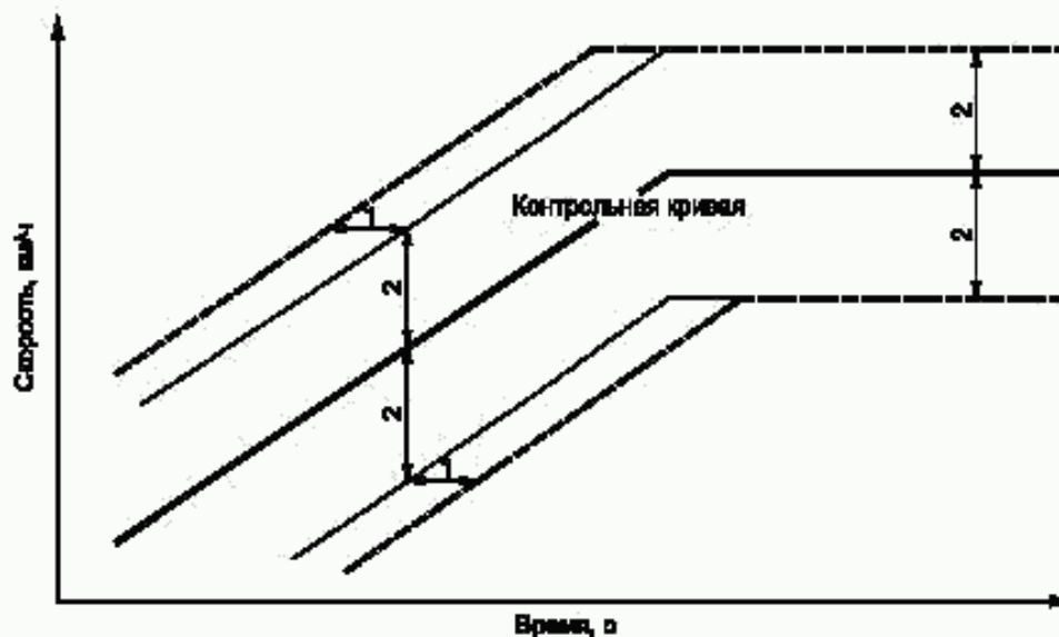
Рисунок 4 — Допустимое отклонение скорости
