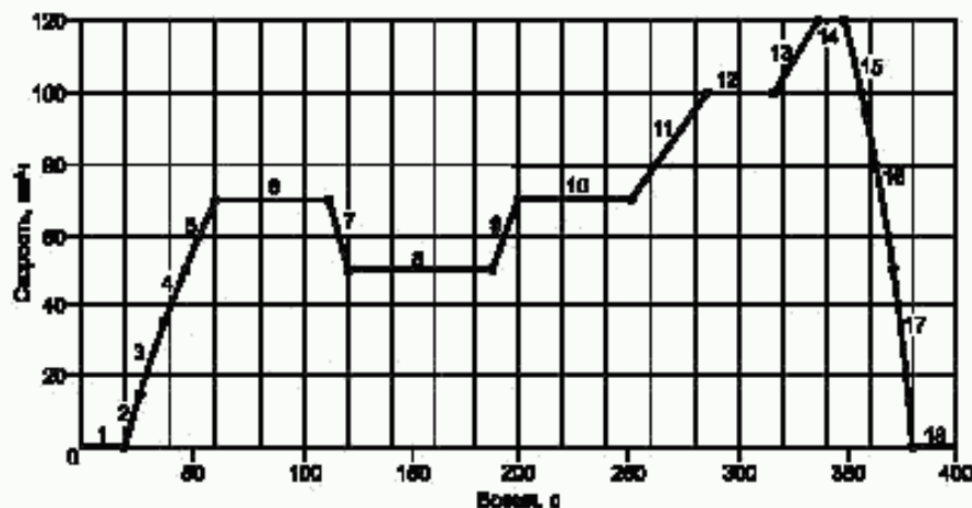
Рисунок 3 — Загородный цикл (400 с)
