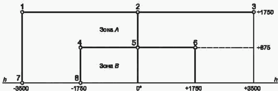
Рисунок 2 — Точки измерения
