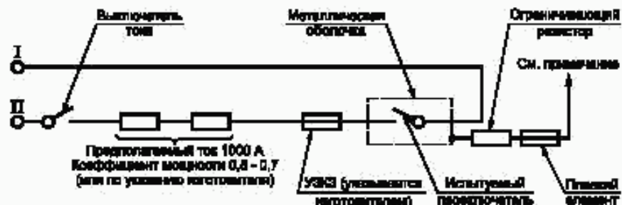
Рисунок 7 — Схема нагрузки L_n для условий испытаний, требующих различных значений токов включения и отключения и/или коэффициентов мощности (постоянной времени)
