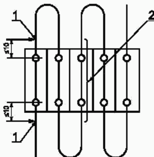
1 — место измерения падения напряжения мультиметром; 2 — место измерения температуры
