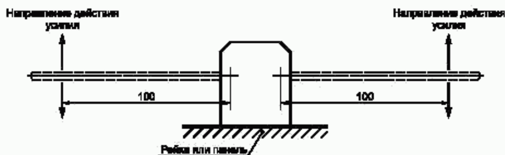
Рисунок 1 — Установка для испытания
