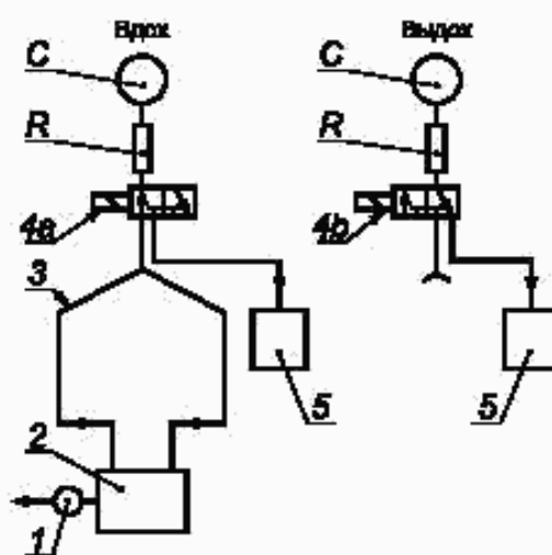
1 — проверяемое устройство для измерения дыхательного объема; 2 — АППАРАТ ИВЛ; 3 — дыхательный контур АППАРАТА ИВЛ; 4а, 4б — пневмораспределитель; 5 — контрольное устройство
