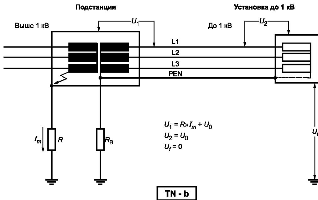
Рисунок 44В — TN-системы
