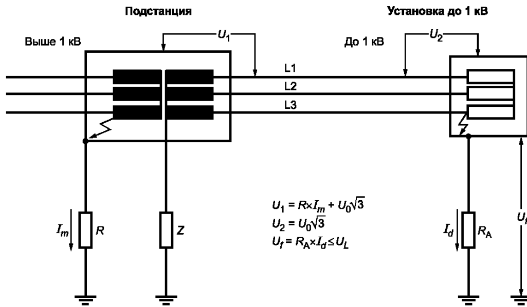
2) Первое замыкание в установке до 1 кВ
