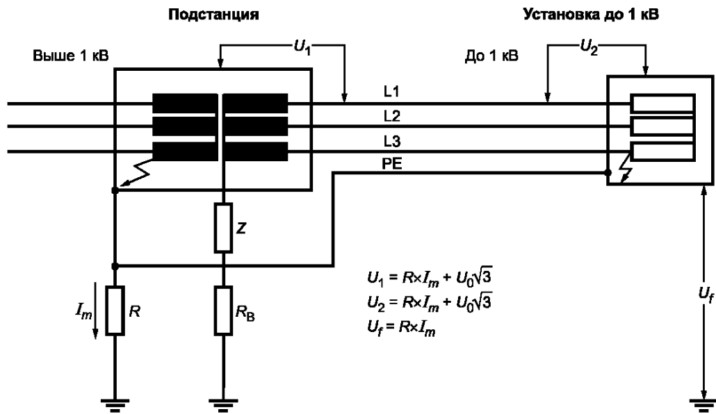
Рисунок 44J — IT-системы, пример e1)
