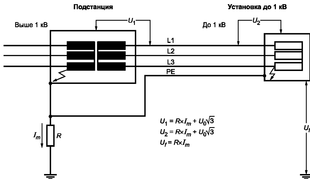
Рисунок 44К — IT-системы, пример е2)
