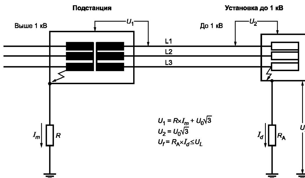
Рисунок 44G — IT-системы, пример с2)
