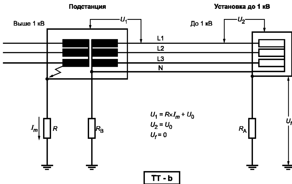
Рисунок 44С — ТТ-системы
