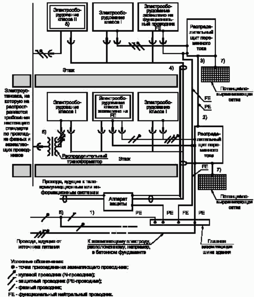
1) — PE-проводник; 2) — распределительный щит; 3) — выравнивание электрических потенциалов; 4) — экранированный провод; 5) — нулевой провод; 6) — разделительный трансформатор; 7) — локальное УВЭП; 8) — электрооборудование
