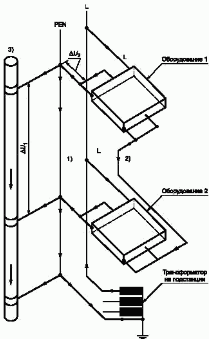
Рисунок 1а — TN-C-система здания
