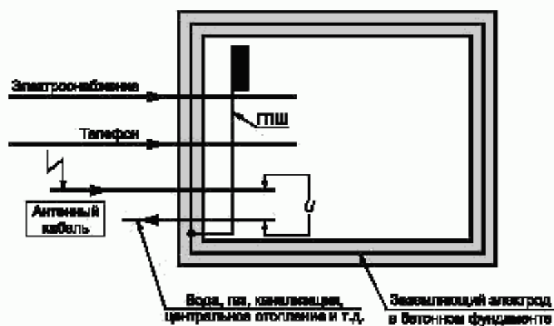
Рисунок 3а — Односторонний ввод (предпочтителен, U = 0 )
