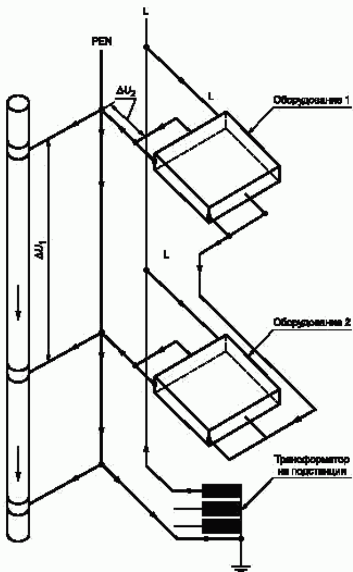
Рисунок 2а — Система заземления типа TN-C
