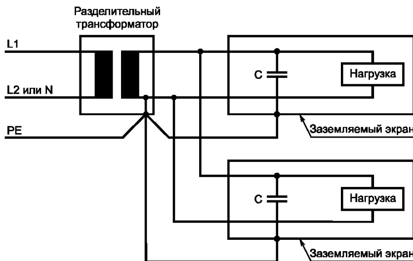
Рисунок А.1 — Границы между электростанцией и оборудованием обработки информации
