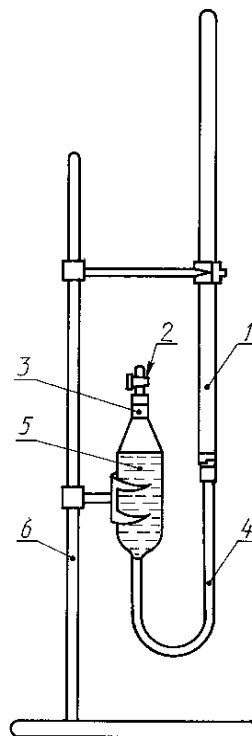
1 — бюретка; 2 — кран; 3 — пробка; 4 — резиновая трубка; 5 — резервуар; 6 — штатив
