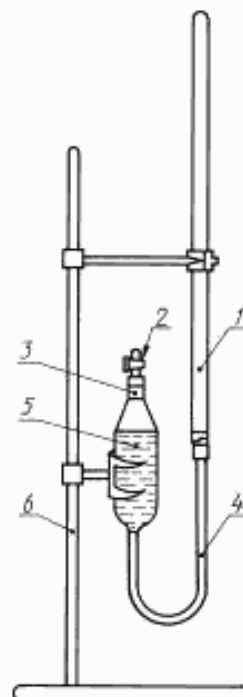
1 — бюретка; 2 — кран; 3 — пробка; 4 — резиновая трубка; 5 — резервуар; 6 — штатив
