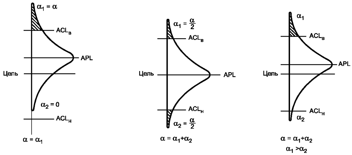
а) случай с обычными требованиями технического допуска
