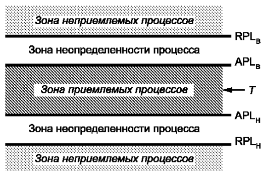
Рисунок 1 — Поле допуска: верхняя и нижняя линии APL и RPL в сопоставлении с зонами приемлемого, неприемлемого процессов и зоной неопределенности процесса
