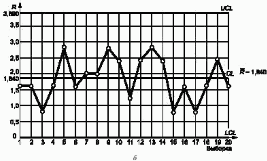
Рисунок Г.2 — Карты средних (а) и размахов (б) по данным таблицы Г.2
