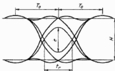
Рисунок 10 — Оциллограмма глазковой диаграммы
