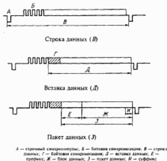
Рисунок 5 — Структура строки данных
