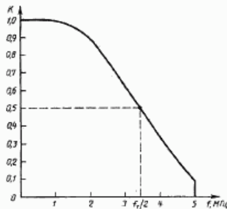
Рисунок 1 — Форма спектра импульсов цифровых данных
