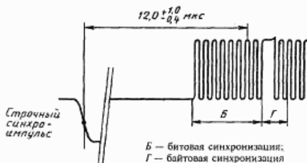
Рисунок 3 — Синхронизация сигнала цифровых данных телетекста
