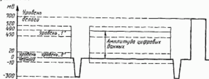
Рисунок 2 — Уровни сигнала цифровых данных сигнала телетекста
