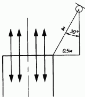
Рисунок А.2 — Измерительные точки у выхлопной или всасывающей трубы
