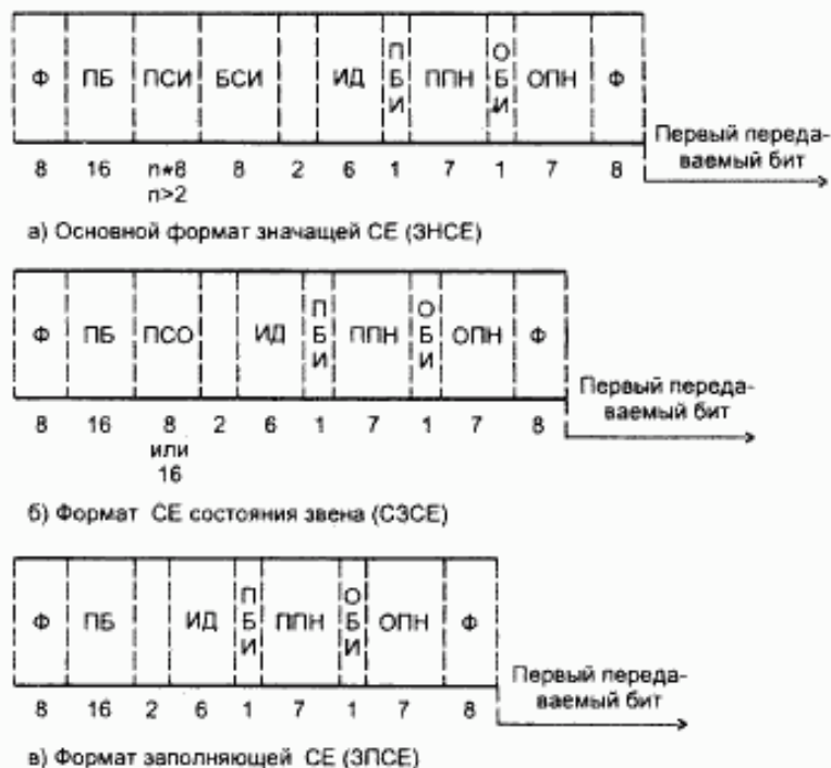
Рисунок 8.2 — Форматы сигнальных единиц
