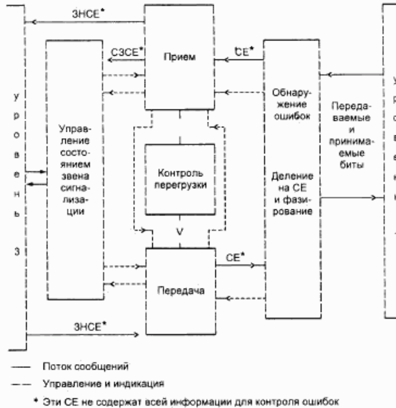
Рисунок 8.1 — Функциональная схема взаимодействия блоков звена сигнализации
