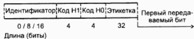
Рисунок 9.4 — Формат сообщений управления сетью сигнализации
