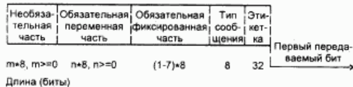
Рисунок 9.3 — Формат сообщений ПУСС
