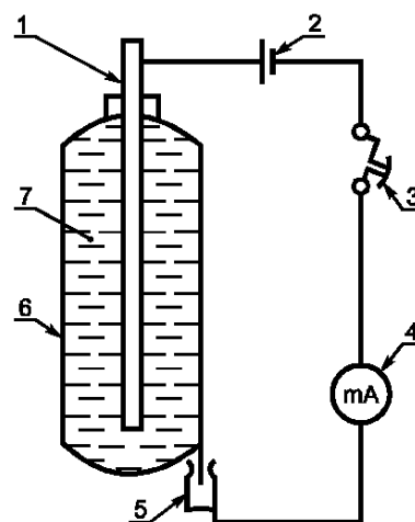
1 — электрод; 2 — стабилизированный источник постоянного тока с напряжением 3,7 В; 3 — выключатель; 4 — миллиамперметр с пределом измерения до 200 мА; 5 — зажим; 6 — корпус огнетушителя; 7 — раствор электролита
