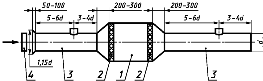
1 — кондиционер; 2 — уплотнение; 3 — измерительная труба; 4 — дозатор пыли (пылешитатель); d — диаметр измерительной трубы
