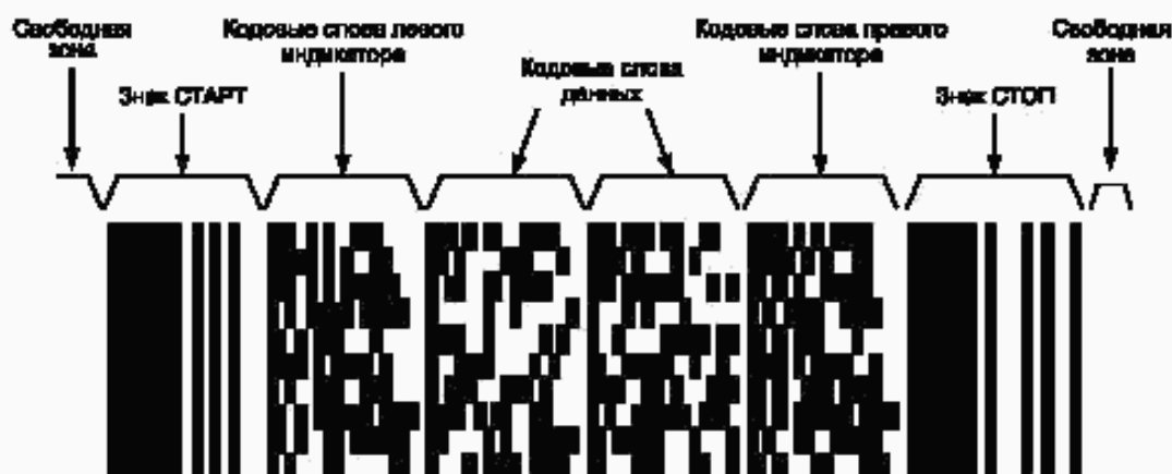
Рисунок 1 — Структура символа PDF417.
