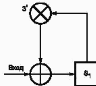
Рисунок L.1 — Делитель синдрома символа
