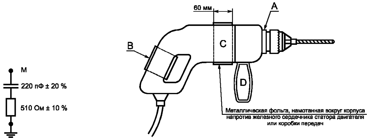
Рисунок 8а — Элемент RC
