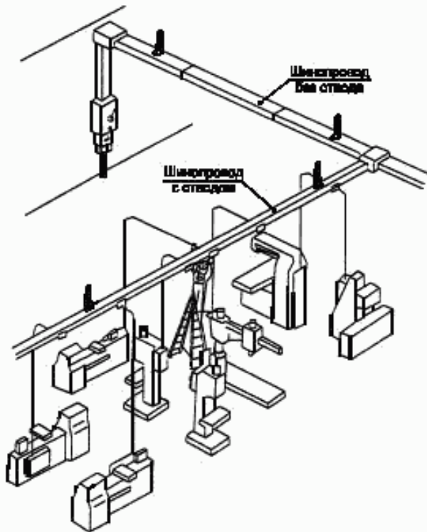
Рисунок С.7 — Система сборных шин (шинопровод)
