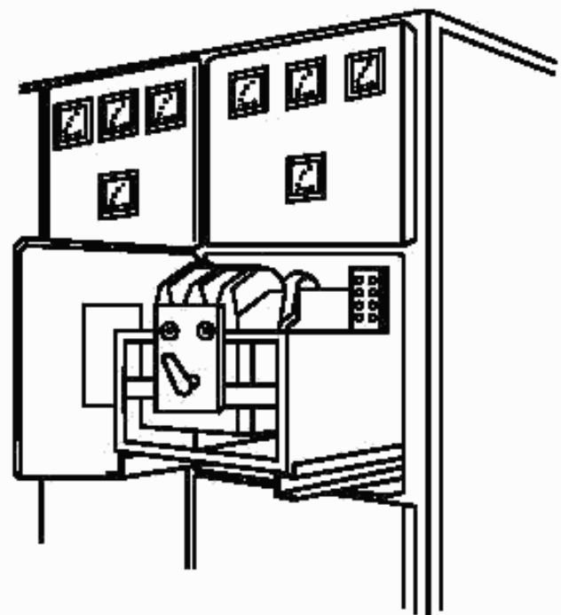
Рисунок С.10 — Выдвижная часть
