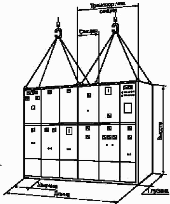
Рисунок С.4 — НКУ заводского изготовления многошкафного типа
