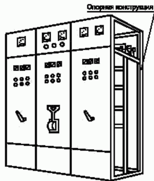
Рисунок С.2 — НКУ заводского изготовления открытого типа, защищенное спереди
