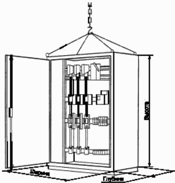
Рисунок С.3 — НКУ заводского изготовления шкафного типа
