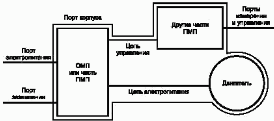
Рисунок 2— Примеры портов СЭП
