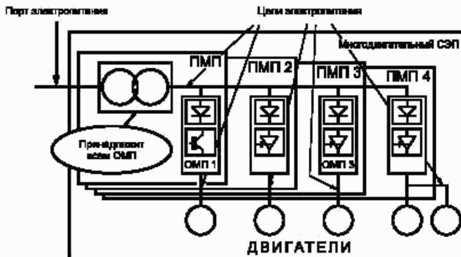
Рисунок 4 — Цепи электропитания СЭП с общим входным трансформатором
