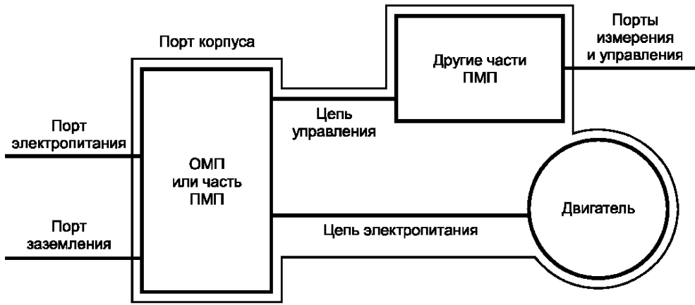
Рисунок 2— Примеры портов СЭП
