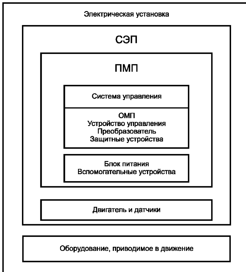
Рисунок 1 — Составные части электрической установки, включающей СЭП
