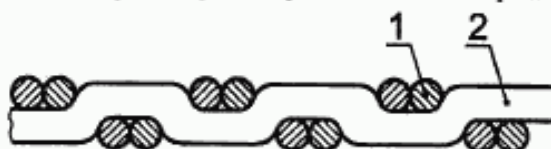
1 — нить основы ворсованная, 2 — нить утка ворсованная
