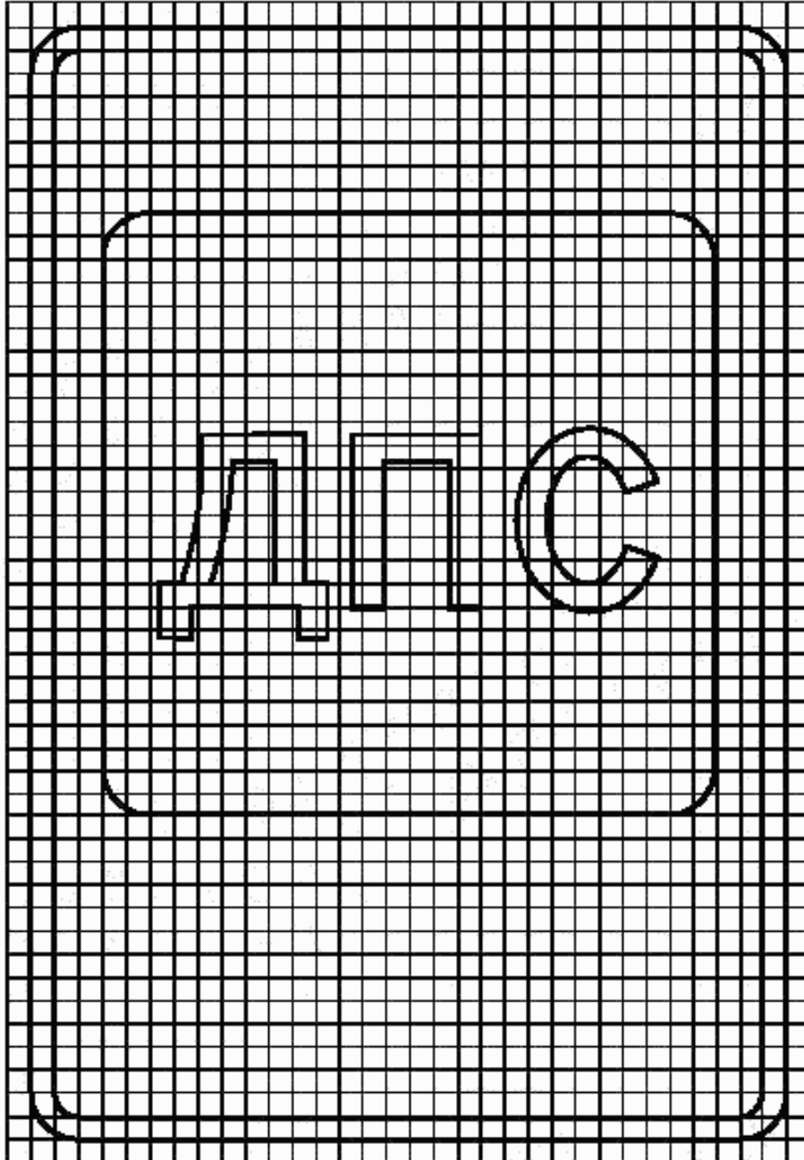
Рисунок Б.2 — Знак 6.14
