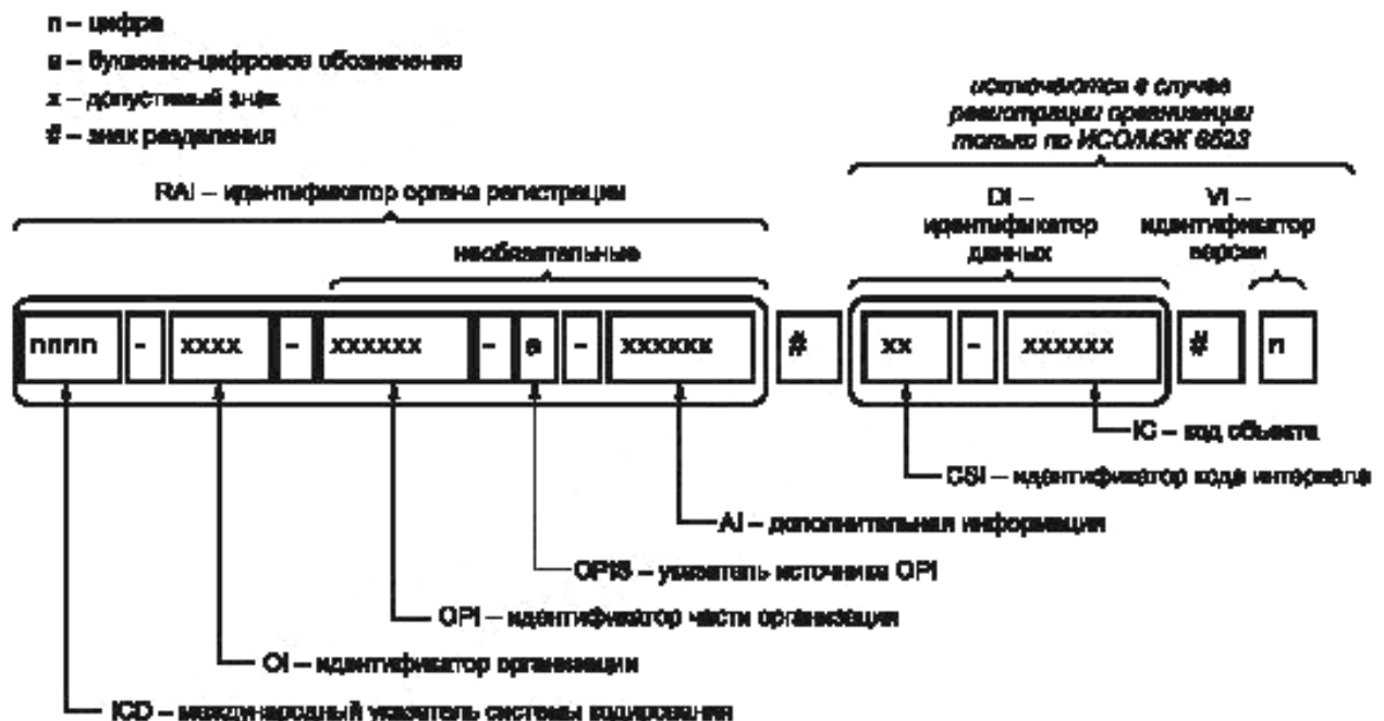
Рисунок 1 — Структура идентификатора IRDI
