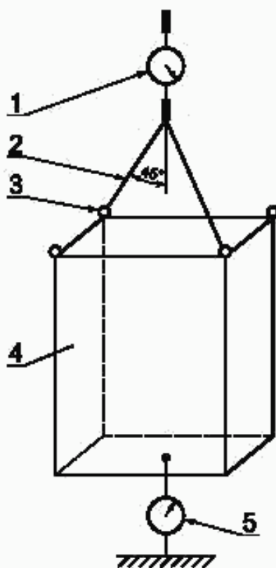
1 — динамометр 1; 2 — строп; 3 — строповое устройство; 4 — ВРУ; 5 — динамометр 2
