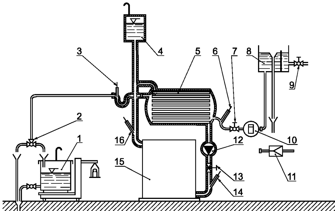
Рисунок И.1 — Испытательный стенд с прямой рециркуляцией
