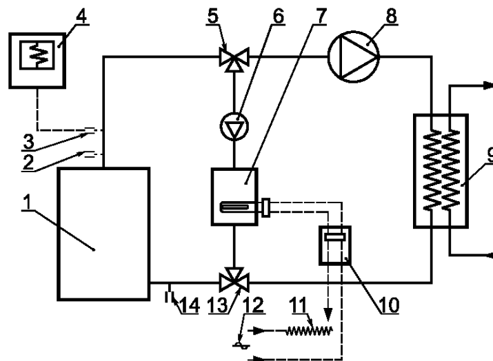
1 — испытуемый котел; 2, 14 — измерители температуры; 3 — термопара; 4 — записывающее устройство; 5, 13 — трехходовые краны; 6 — циркуляционный насос; 7 — электрический водонагреватель; 8 — дополнительный насос (при необходимости); 9 — теплообменник; 10 — электрический счетчик; 11 — регулятор напряжения; 12 — подвод электропитания
