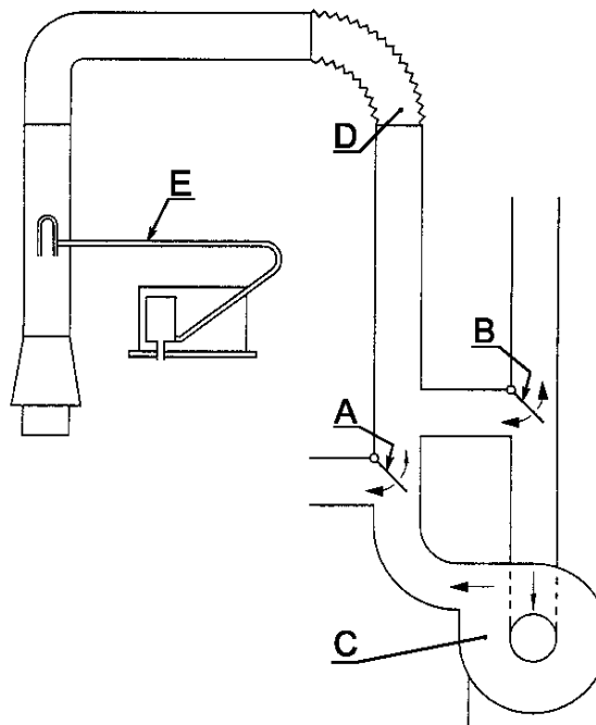
Рисунок И.5 — Испытание котла при особых условиях тяги
