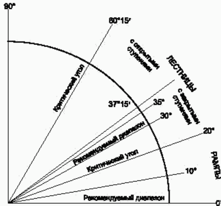
Рисунок 1 — Углы наклона средств доступа к рабочему месту
