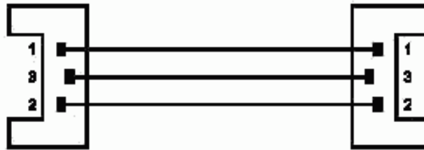
Рисунок Е.2 — Схема соединений кабеля шины
