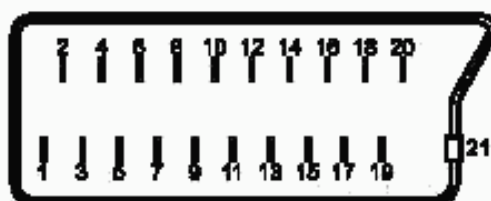
Рисунок В.1 — Расположение и нумерация контактов соединителя
