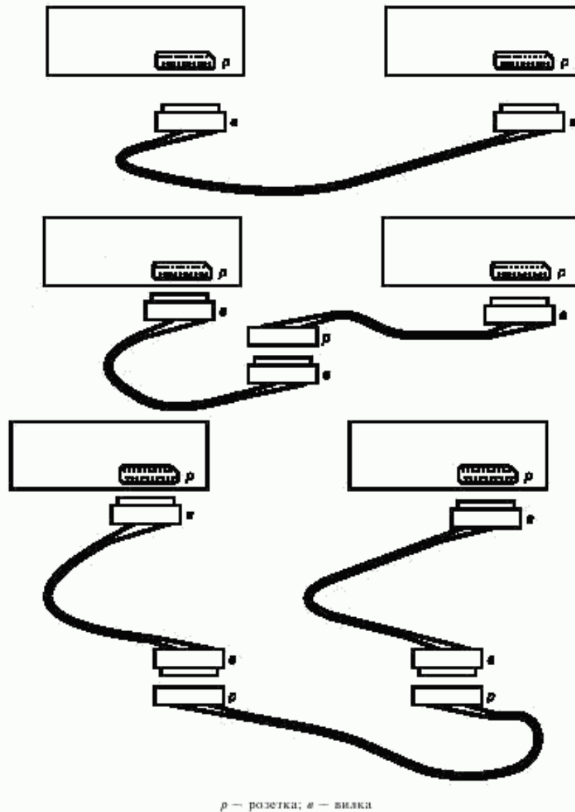
Рисунок В.2 — Виды соединительных шнуров
