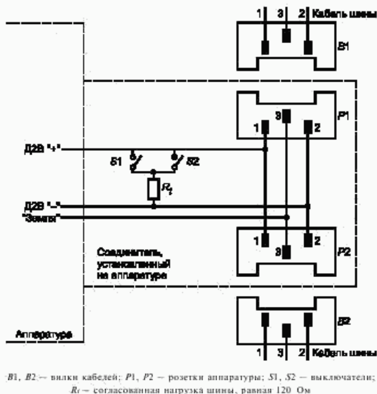
Рисунок Е.1 — Схема подключения аппаратуры к шине Д2В
