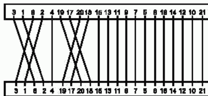
Рисунок В.3 — Кросс-соединения в шнурах аппаратуры с одинаковыми типами соединителей на концах шнура
