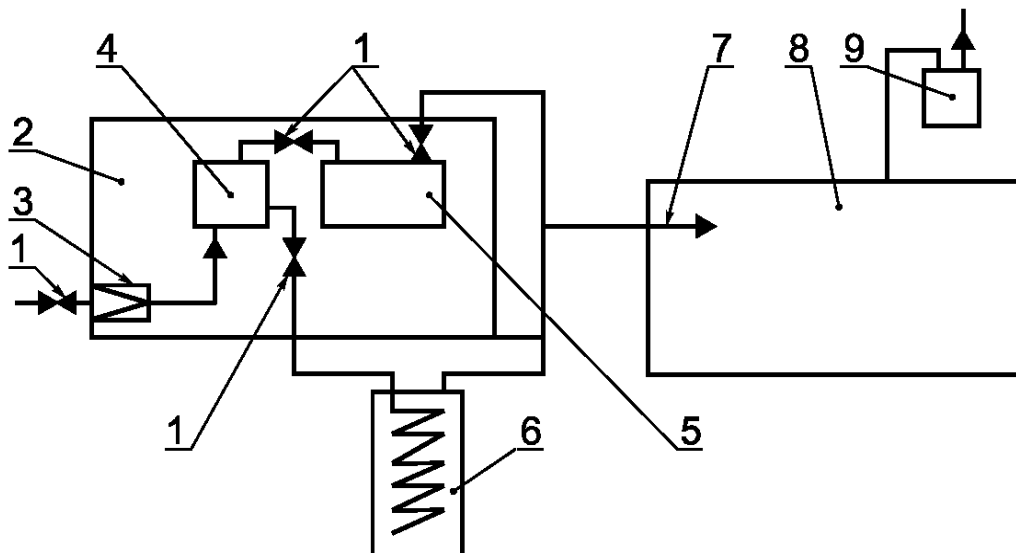
1 — вентиль двухходовой; 2 — камера испарителя; 3 — редуктор; 4 — ресивер; 5 — емкость испарителя; 6 — увлажнитель воздуха; 7 — форсунка; 8 — испытательная камера; 9 — электровентиль
