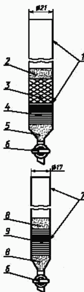
1 — колонка 1 (щелочная) длиной 250 мм; 2 — хлопковая вата или стекловата; 3 — смесь диатомовой земли и анализируемого образца; 4 — 3 г диатомовой земли и 2 см 3 NaOH (5,16 г); 5 — хлопковая вата или стекловата; 6 — кран, предпочтительно из политетрафторэтилена; 7 — колонка 2 (кислотная) длиной 250 мм; 8 — стекловата; 9 — 3 г диатомовой земли и 3 см 3 H 2 SO 4 (6,36 г)
